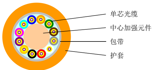
多芯分支室内光缆 I 型
